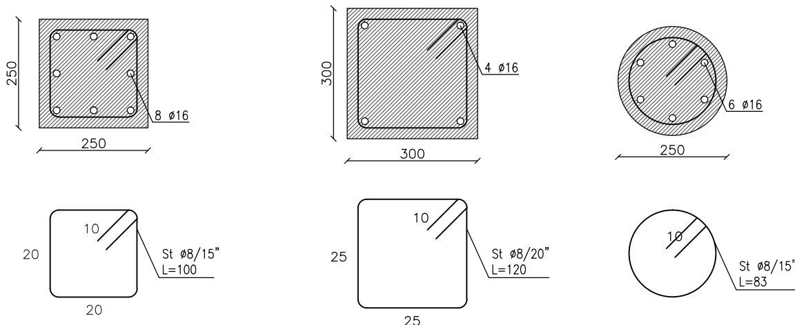
Pilastri H max=100 cm
