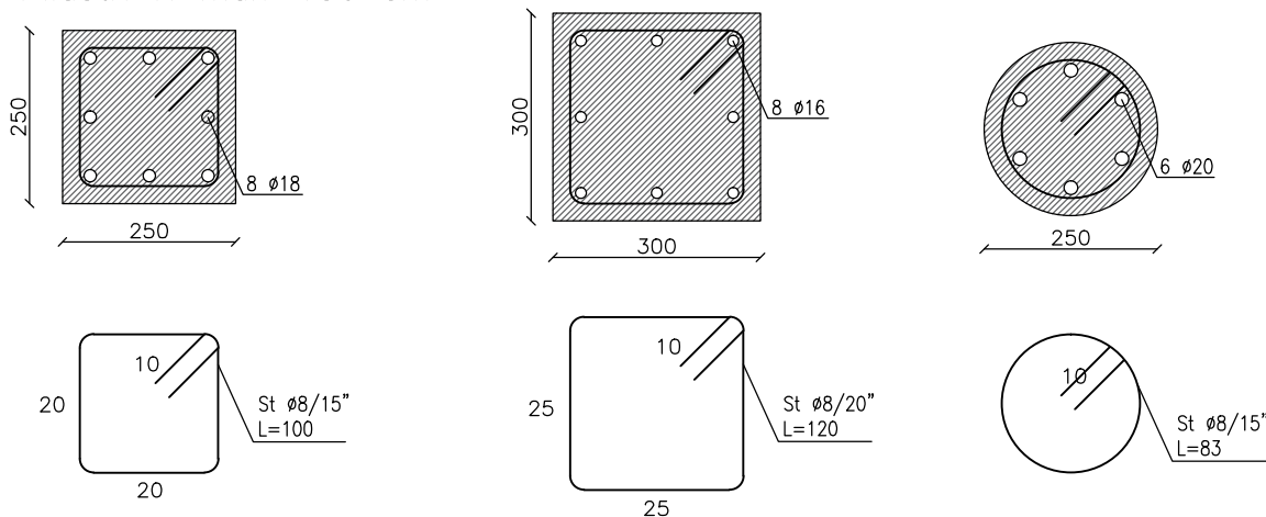
Pilastri H max=150 cm
