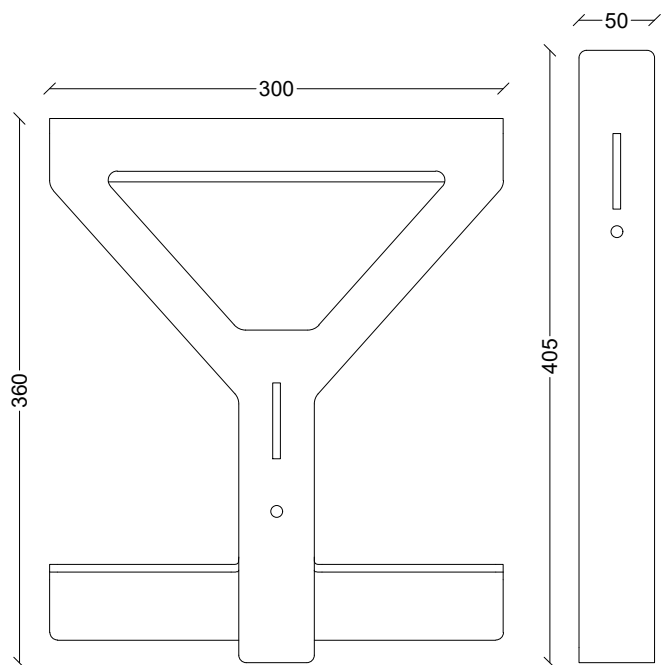
VISTA FRONTALE
